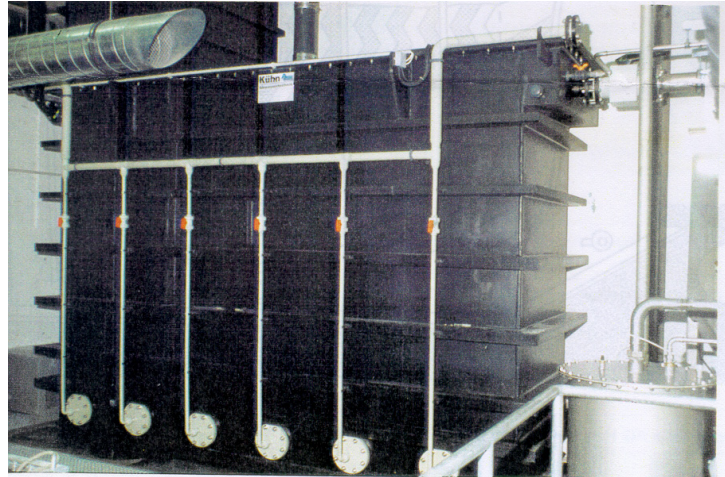
Festbettreaktor zur biologischen Reinigung
